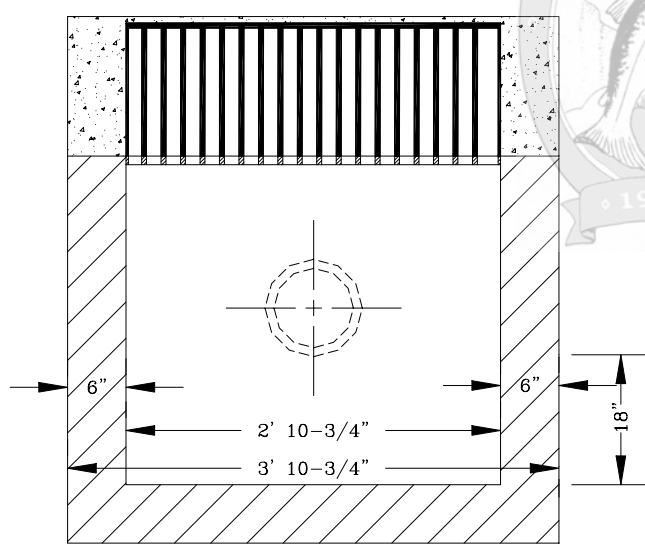
ELEVATION A-A
