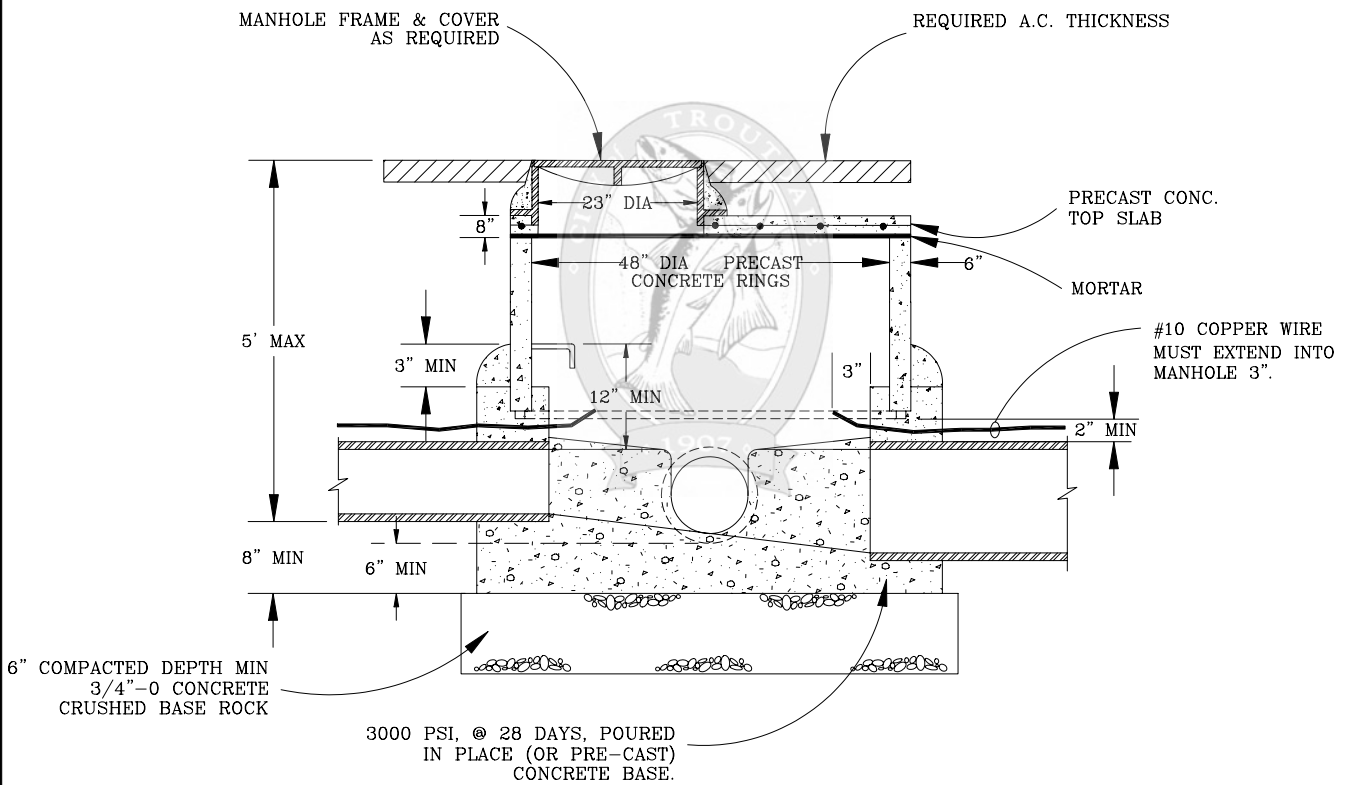
SECTION A-A
